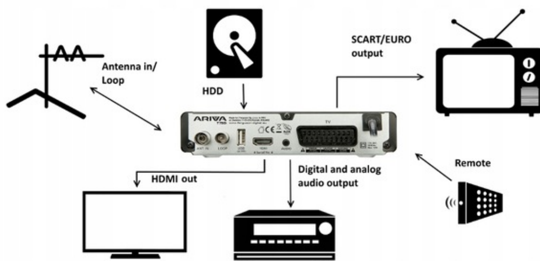
Schemat ilustracyjny przedstawiający zastosowanie tunera:
