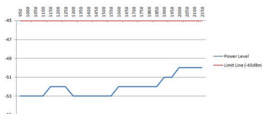
TEST INTERFERENCJI LNB SINGLE GT-SAT GT-S40M:
