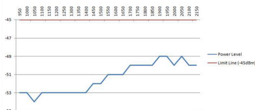
TEST INTERFERENCJI LNB QUAD GT-SAT GT-QD40M:
