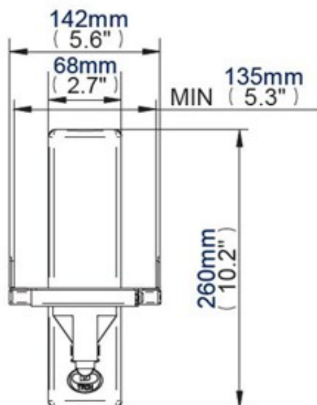
Widok z przodu - minimalny rozstaw
