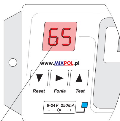
Częstotliwość różnicowa fonii
