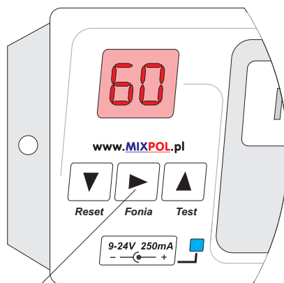
Przycisk zmiany podnośnej fonii
