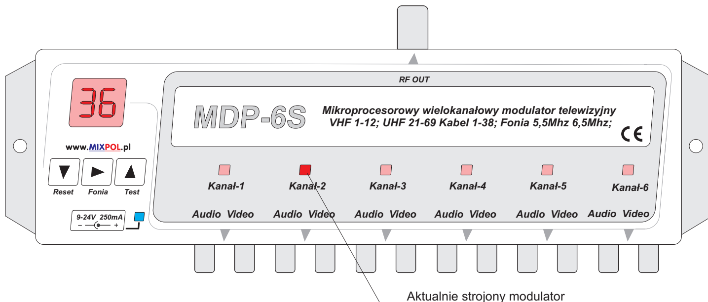
Sygnał testu włączony
